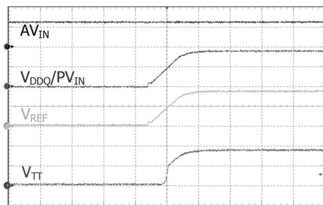
AVIN : 2.0V/div, VDDQ/PVIN : 1.0V/div, VREF : 500mV/div, VTT : 500mV/div, Time : 10ms/div
