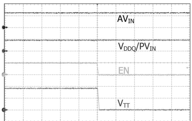
AVIN : 2.0V/div, VDDQ/PVIN : 2.0V/div, EN : 2.0V/div, VTT : 500mV/div, Time : 10ms/div
