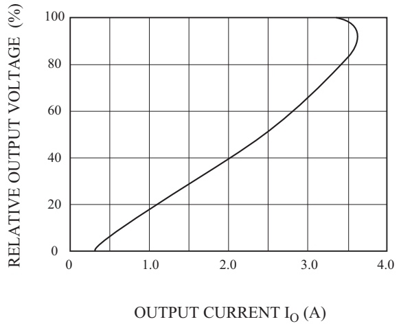
Fig.4 I_O - V_O
