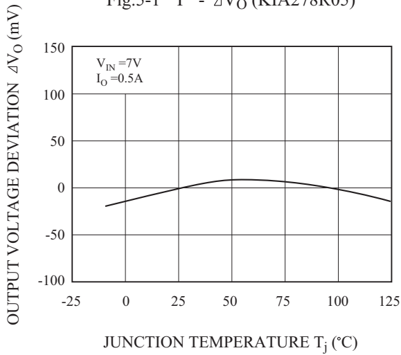
Fig.5-1 T - \Delta V_O (KIA278R05)
