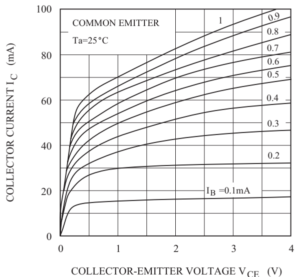
I_C - V_{CE}
