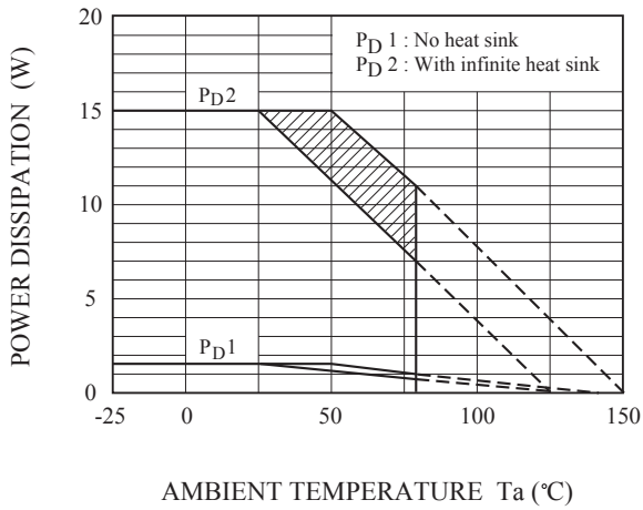
Fig. 3 T_a - P_D
