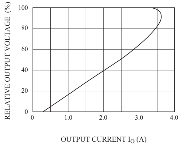
Fig. 4 I_O - V_O
