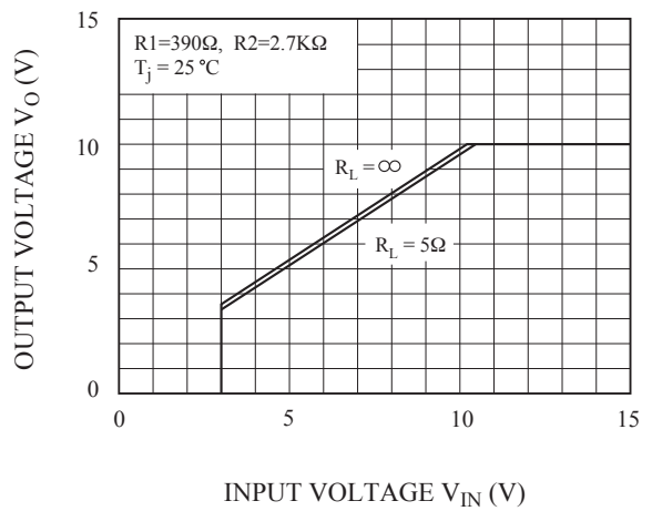
Fig. 6 V_{IN} - V_{OUT}
