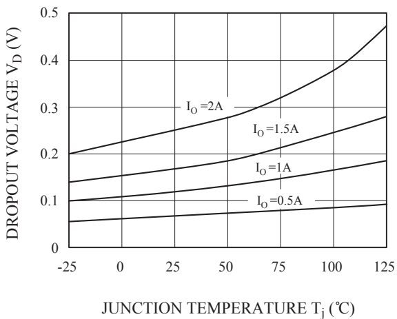
Fig. 7 T_j - V_D
