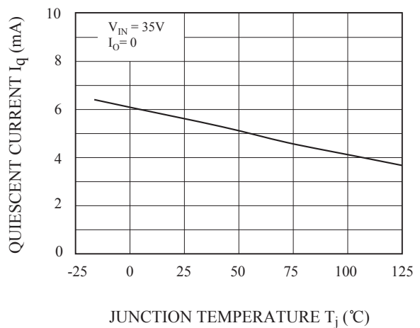
Fig. 8 T_j - I_q
