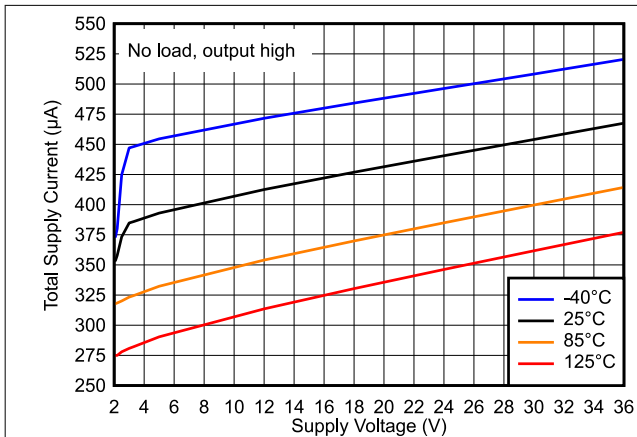
图 6-6. 总电源电流与电源电压之间的关系
