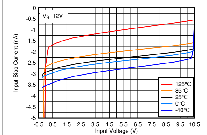
图 6-22. 12V 下输入偏置电流与输入电压之间的关系
